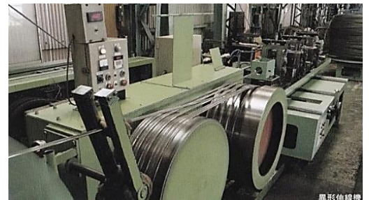
伸線機
